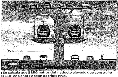
Se calcula que 5 kilómetros del viaducto elevado que construirá el GDF en Santa Fe sean de triple nivel.
